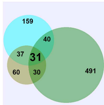
Aquamin (3.0mM)
