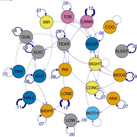
A. UMD
