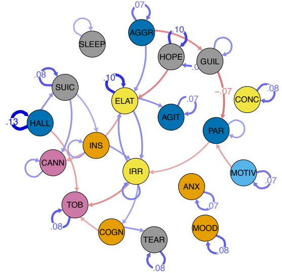
B. BMD
