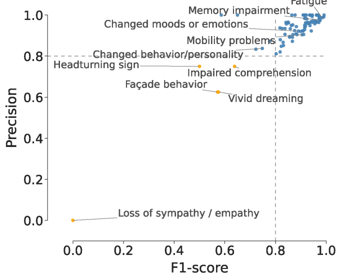
3I T5
