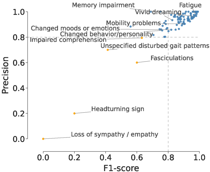
3I T5
