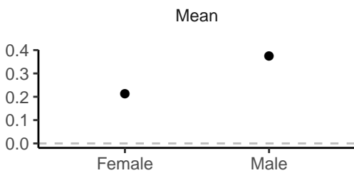
Urate SLC2A9 (rs938555) Sex
