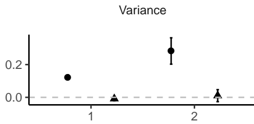
LDL APOE (rs1065853) Sex
