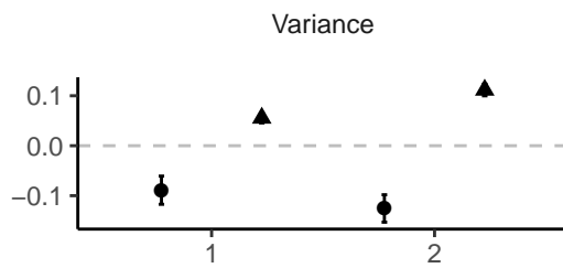
Urate SLC2A9 (rs938555) Sex
