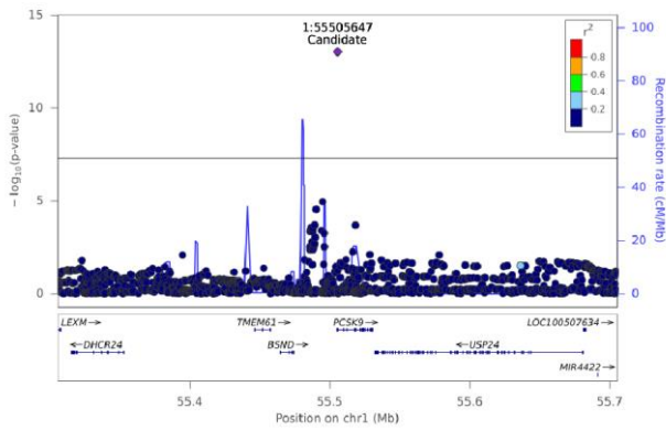
CE(18:1) - Chr 1 (55305731-55705623)
