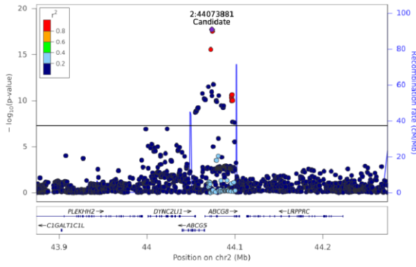
CE(24:4) - Chr 2 (43874118-44273800)
