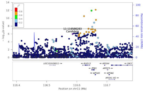
DG(18:1_18:2) - Chr 11 (116386360-116785341)
