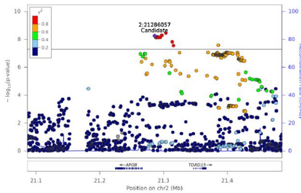
PC(38:2) - Chr 2 (21086225-21485848)
