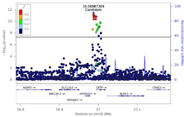
PC(O-32:1) - Chr 16 (56787882-57185761)
