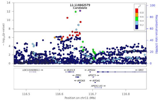
CE(22:0) - Chr 11 (116462788-116862245)
