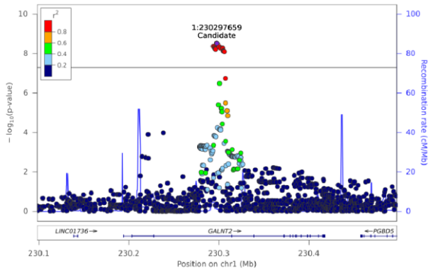
DG(18:1_18:1) - Chr 1 (230097883-230497633)
