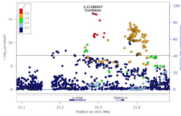
PC(16:0_18:0) - Chr 2 (21086225-21485848)
