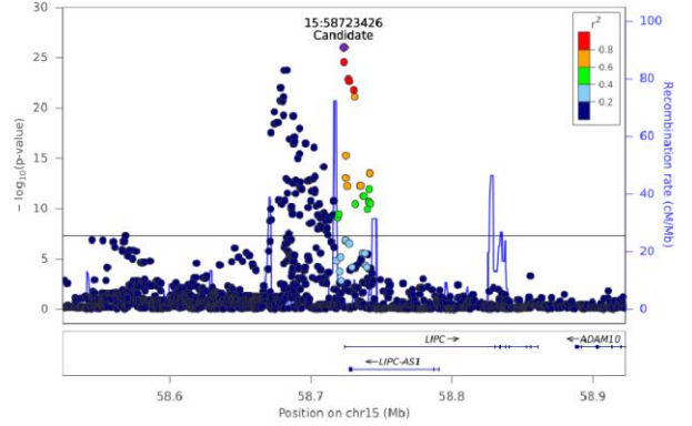
PE(15-MHDA_20:4) - Chr 15 (58524080-58923206)
