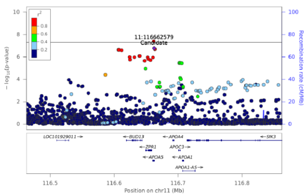
PE(18:1_18:2) - Chr 11 (116462788-116862245)
