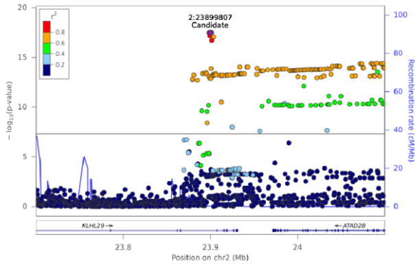
AC(18:1) - Chr 2 (23700054-24099798)
