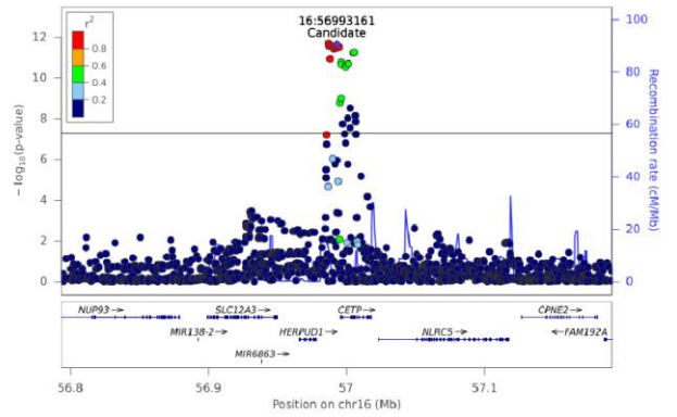
PC(O-40:7) (a) - Chr 16 (56793346-57192310)
