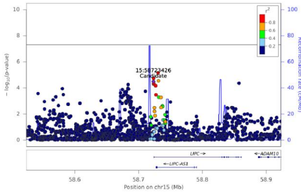
PE(15-MHDA_22:6) - Chr 15 (58524080-58923206)
