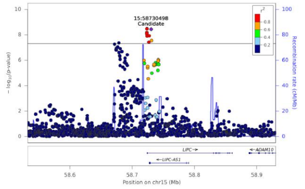
PC(18:1_18:1) - Chr 15 (58532076-58930416)
