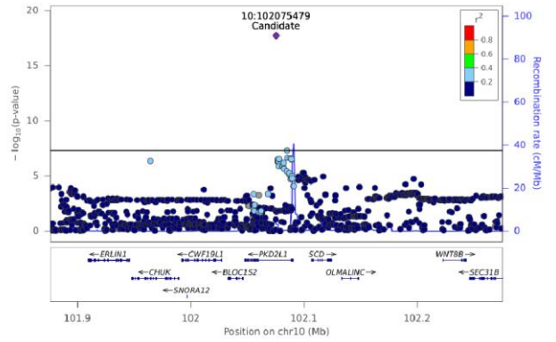
AC(16:1) - Chr 10 (101875936-102275471)
