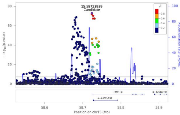
PE(18:0_20:4) - Chr 15 (58524080-58923790)
