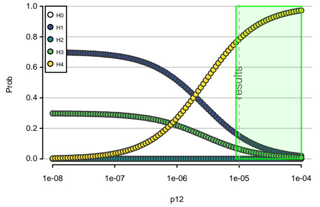
Posterior probabilities
