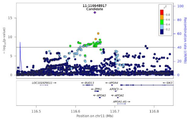
DG(18:1_18:3) - Chr 11 (116448927-116848857)
