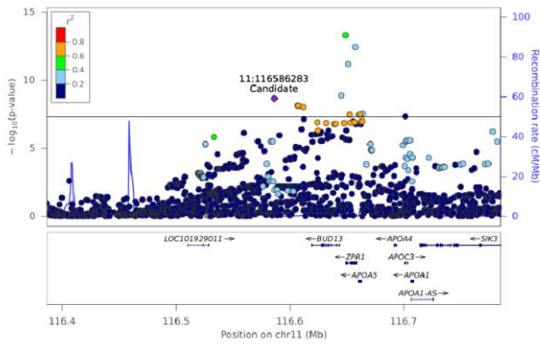
CE(16:2) - Chr 11 (116386360-116785341)
