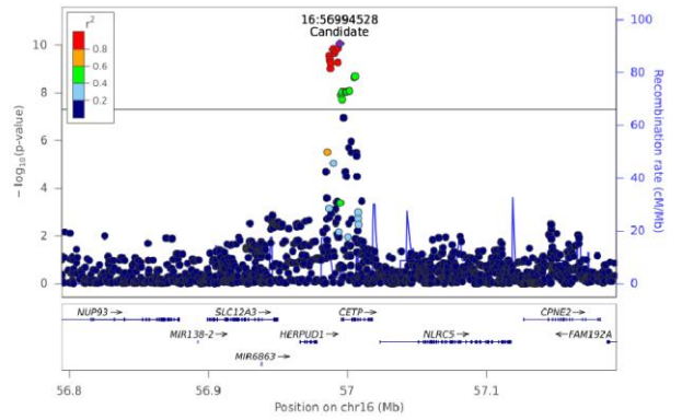
PC(O-34:1) - Chr 16 (56794590-57193448)
