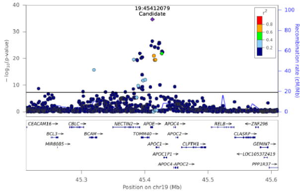
CE(16:0) - Chr 19 (45212381-45610846)
