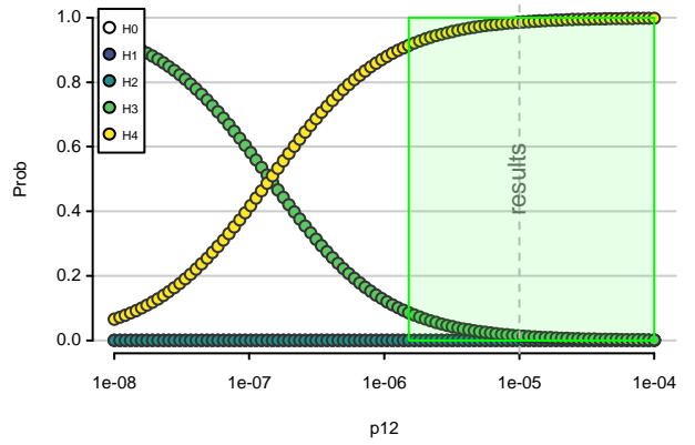
Posterior probabilities
