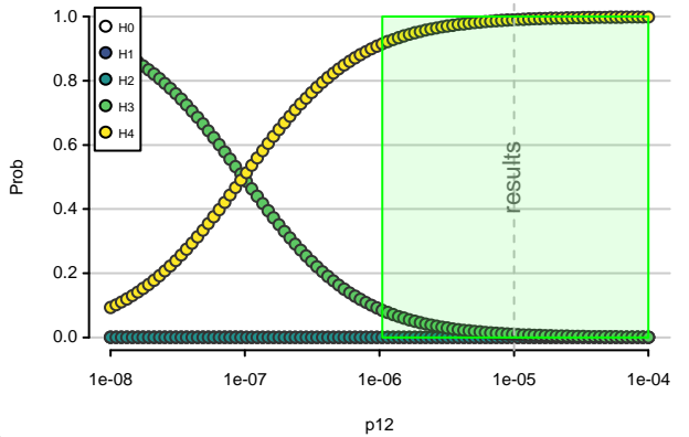
Posterior probabilities
