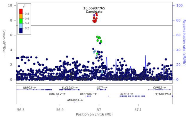
CE(18:0) - Chr 16 (56787882-57187761)
