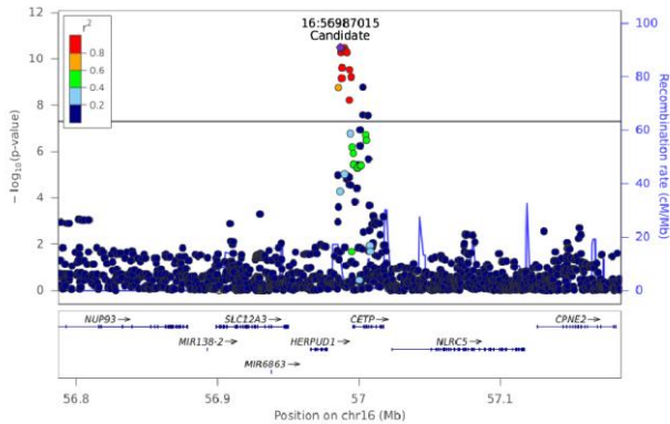
PC(16:0_18:3) (b) - Chr 16 (56787107-57185761)
