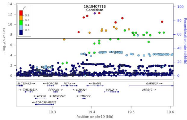
DG(18:2_20:4) - Chr 19 (19208076-19607564)
