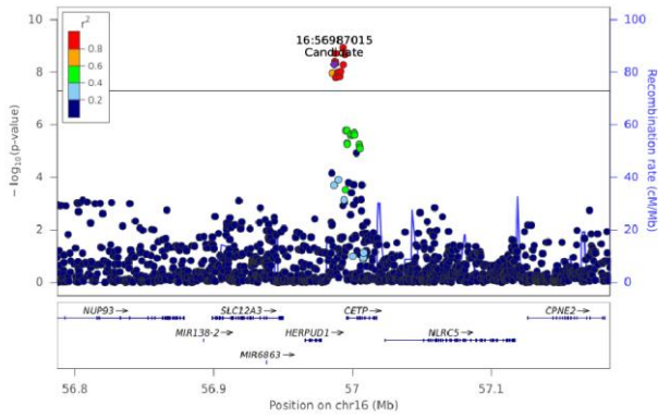
PC(16:0_16:0) - Chr 16 (56787107-57185761)
