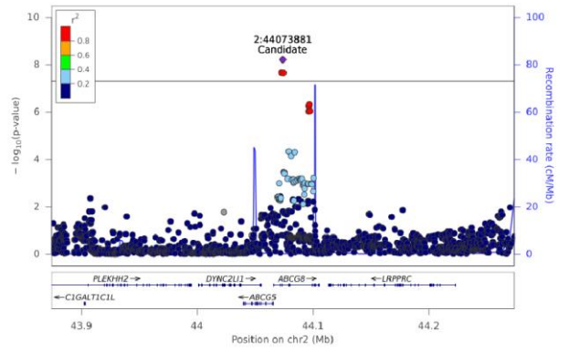
CE(24:5) - Chr 2 (43874118-44273800)
