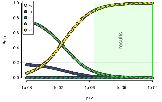
Posterior probabilities
