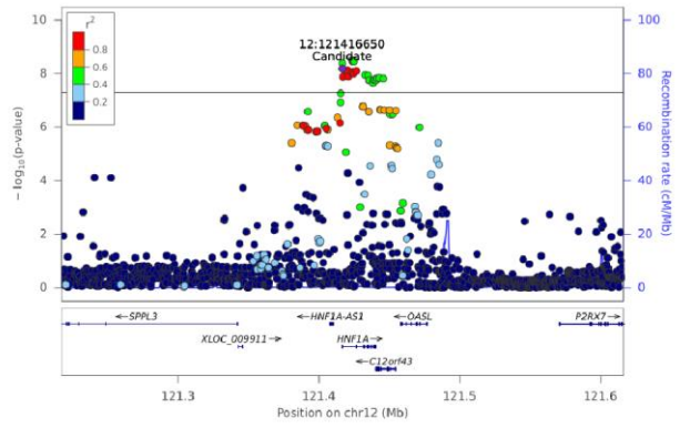
Cer(d17:1/24:1) - Chr 12 (121216911-121616464)
