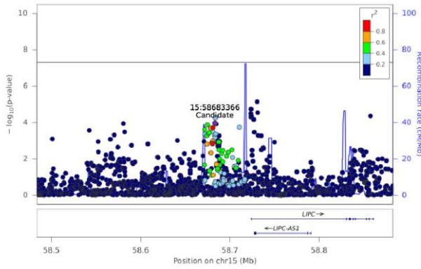
PE(18:1_18:2) - Chr 15 (58483611-58882792)
