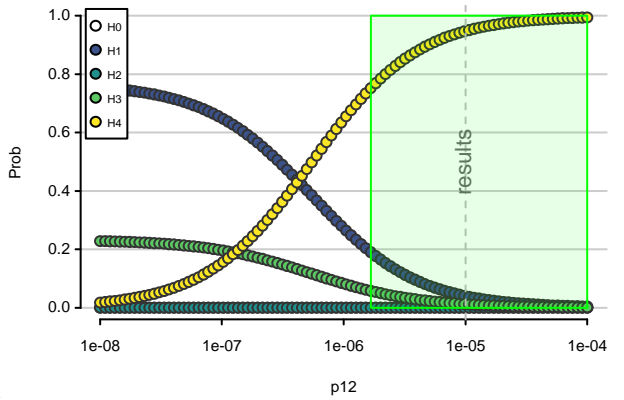
Posterior probabilities
