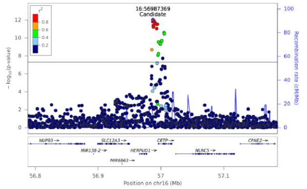
PC(P-16:0/18:1) - Chr 16 (56787882-57185761)
