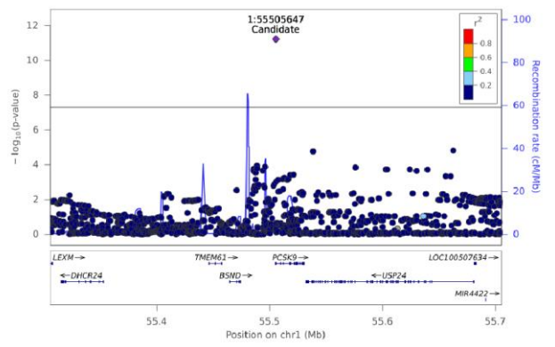
CE(16:0) - Chr 1 (55305731-55705623)
