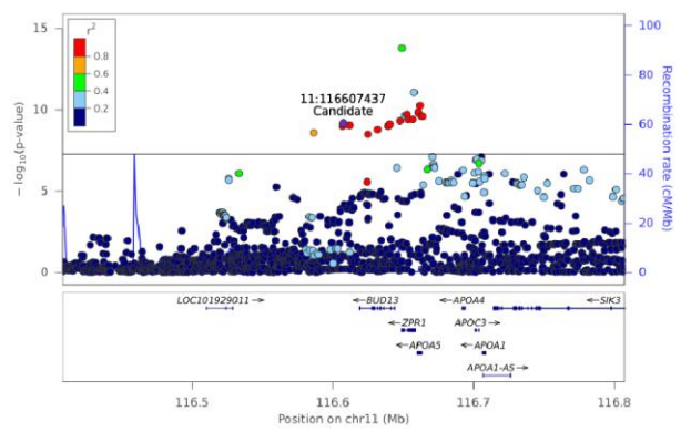
CE(16:1) - Chr 11 (116407583-116807368)
