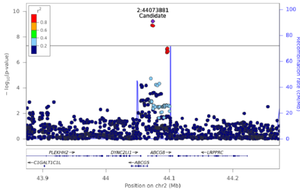
CE(24:1) - Chr 2 (43874118-44273800)
