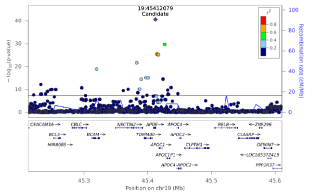
CE(18:1) - Chr 19 (45212381-45610846)
