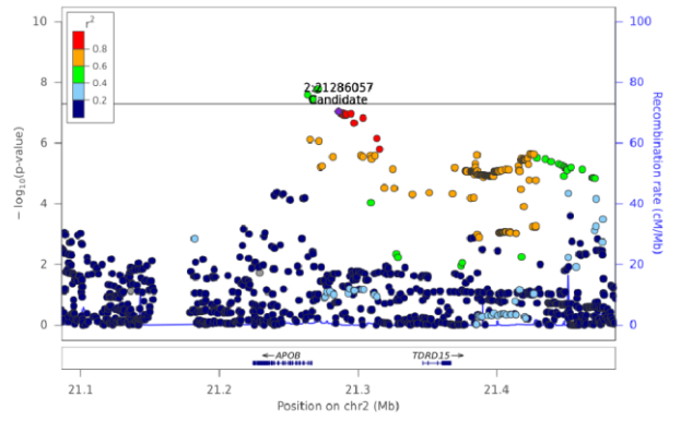
CE(20:2) - Chr 2 (21086225-21485848)
