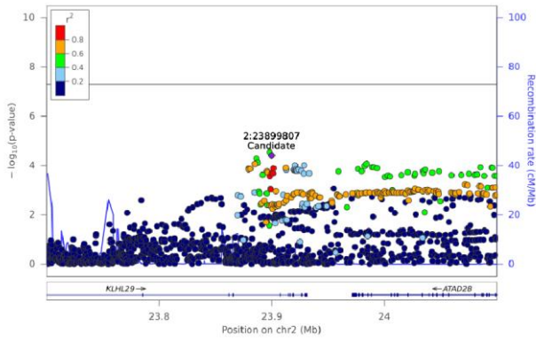
AC(16:0) - Chr 2 (23700054-24099798)
