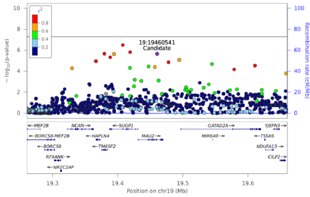
Cer(d18:1/24:0) - Chr 19 (19260686-19660523)
