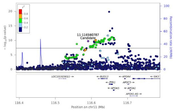
CE(22:6) - Chr 11 (116391073-116789849)
