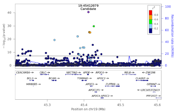
CE(18:2) - Chr 19 (45212381-45610846)
