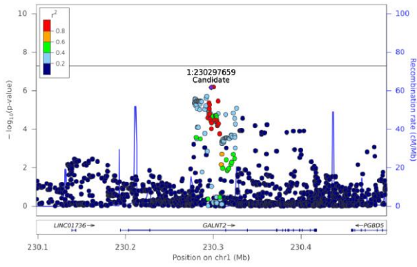
DG(18:0_18:1) - Chr 1 (230097883-230497633)
