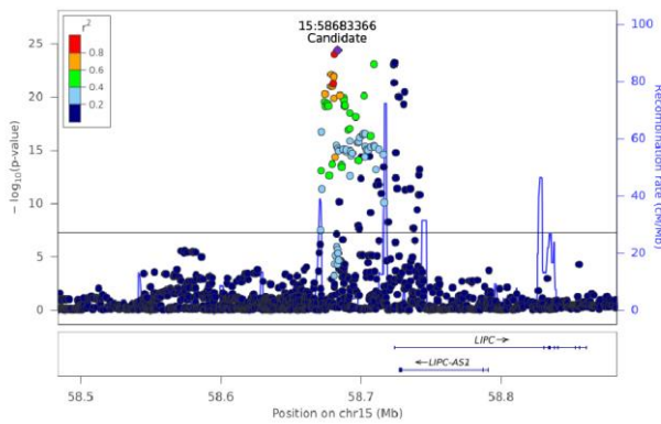
PE(16:0_16:0) - Chr 15 (58483611-58882792)
