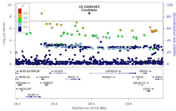
Cer(d18:1/24:1) - Chr 19 (19295556-19693426)
