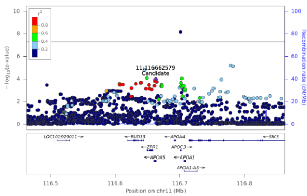
PE(18:1_18:2) - Chr 11 (116462788-116862245)
