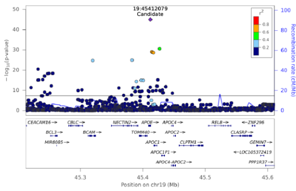
CE(18:2) - Chr 19 (45212381-45610846)
