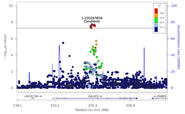
Total DG - Chr 1 (230097883-230497633)
