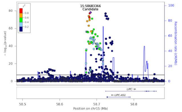
PE(16:0_18:2) - Chr 15 (58483611-58882792)
