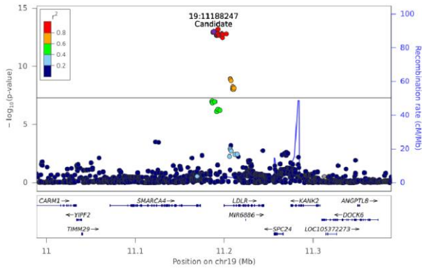
SM(d18:1/16:0) - Chr 19 (10988818-11388151)
