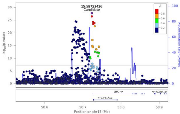
PE(18:0_20:3) (b) - Chr 15 (58524080-58923206)
