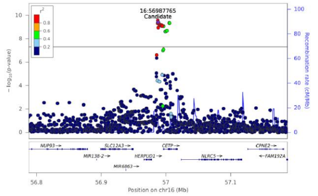
PC(O-16:0/16:0) - Chr 16 (56787882-57187761)
