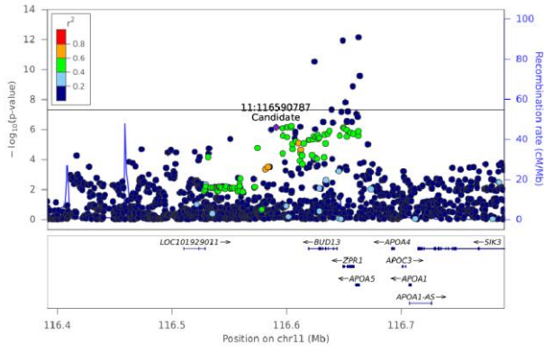
DG(18:0_18:1) - Chr 11 (116391073-116789849)
