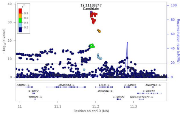
Total SM - Chr 19 (10988818-11388151)
