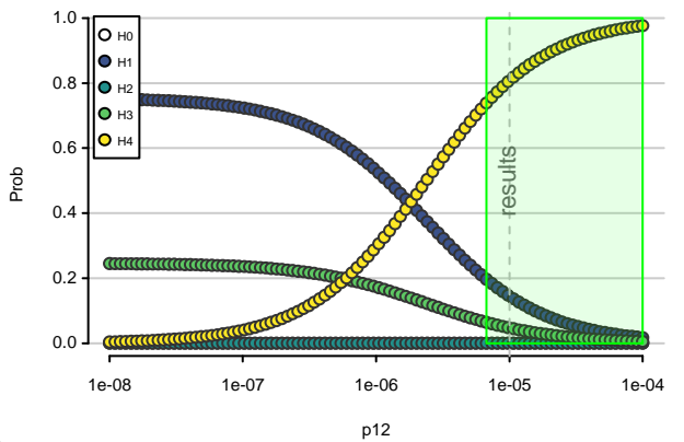
Posterior probabilities
