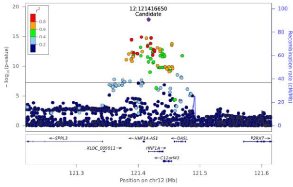
Cer(d18:2/24:1) - Chr 12 (121216911-121616464)
