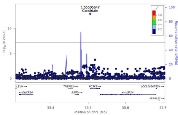
CE(18:1) - Chr 1 (55305731-55705623)
