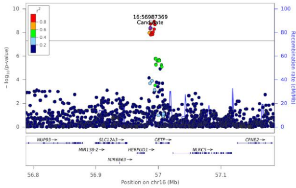
PC(P-16:0/16:1) - Chr 16 (56787882-57185761)
