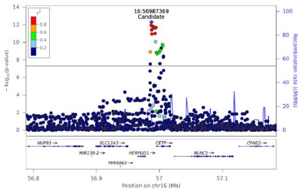
PC(O-32:1) - Chr 16 (56787882-57185761)
