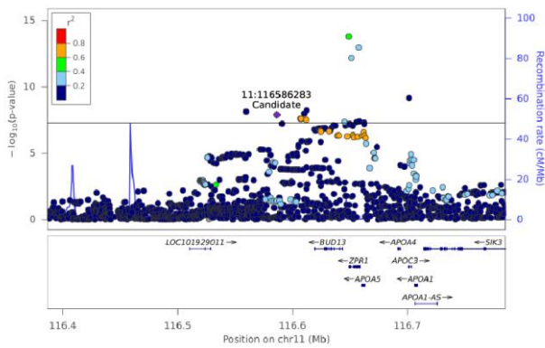
CE(16:2) - Chr 11 (116386360-116785341)
