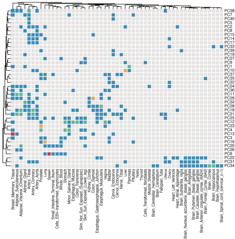
a GTEx v7
