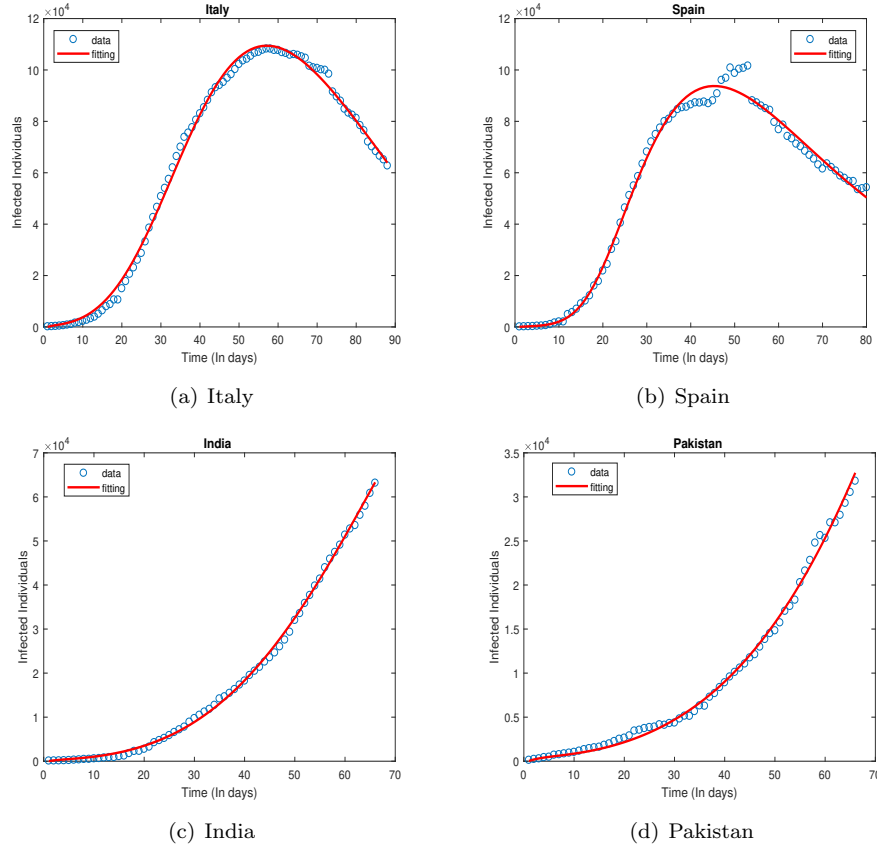
Figure 6: Parameter Estimation
