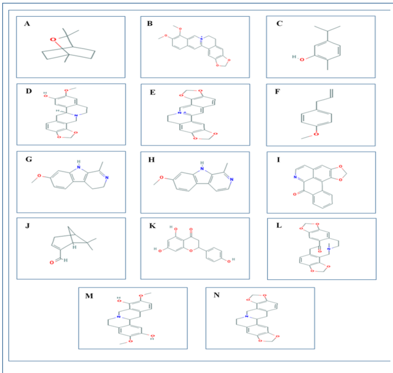
Figure 04. 2D representations of the all the 14 ligands used in the experiment. The ligand structures were taken from PubChem server ( www.pubchem.ncbi.nlm.nih.gov ). A. 1,8-cineol (PubChem CID: 2758); B. Berberine (PubChem CID: 2353); C. Carvacrol (PubChem CID: 10364); D. Cheilanthifoline (PubChem CID: 440582); E. Coptisine (PubChem CID: 72322); F. Estragole (PubChem CID: 8815); G. Harmaline (PubChem CID: 3564); H. Harmine (PubChem
