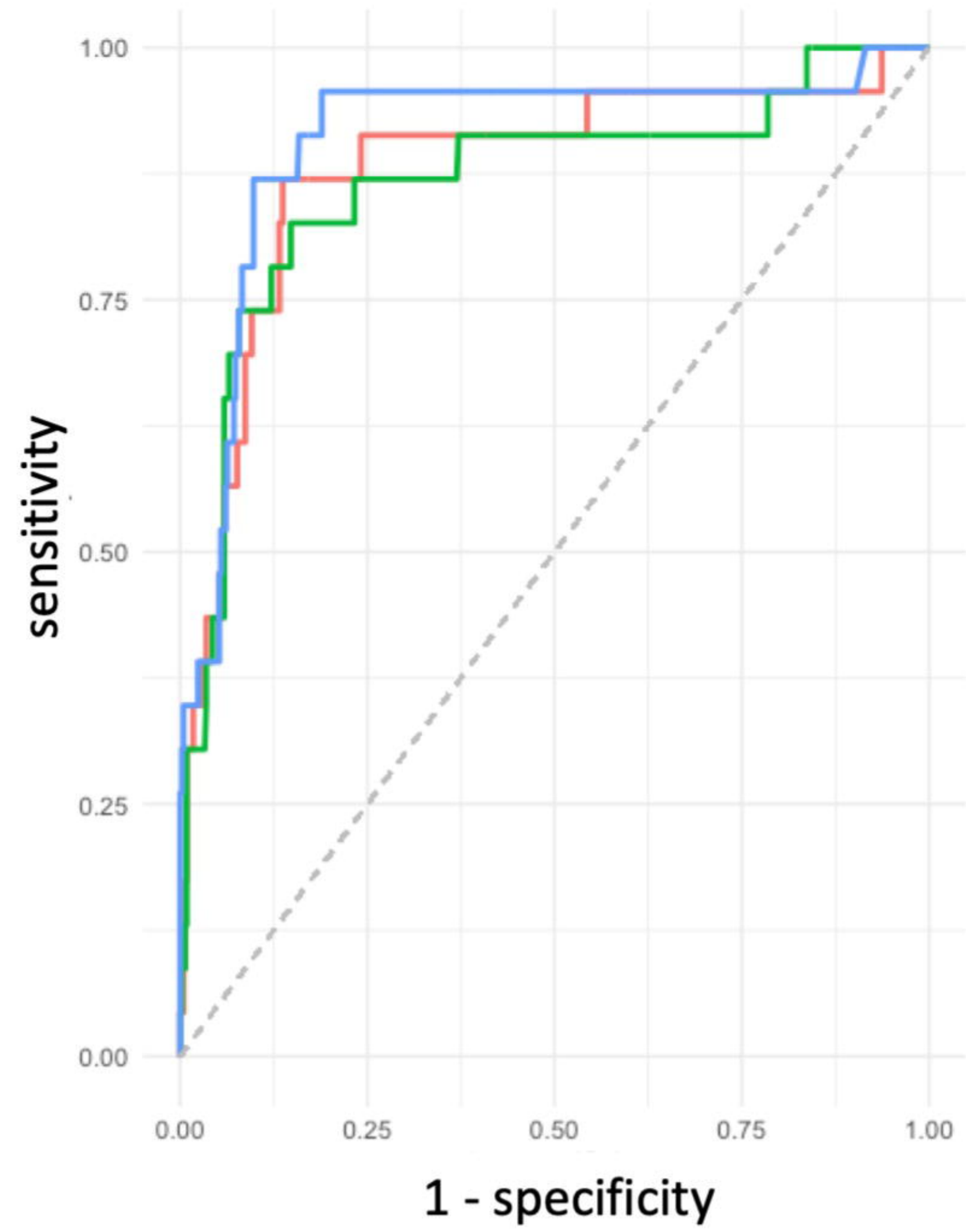
AUC ROC: All prevalent TB
