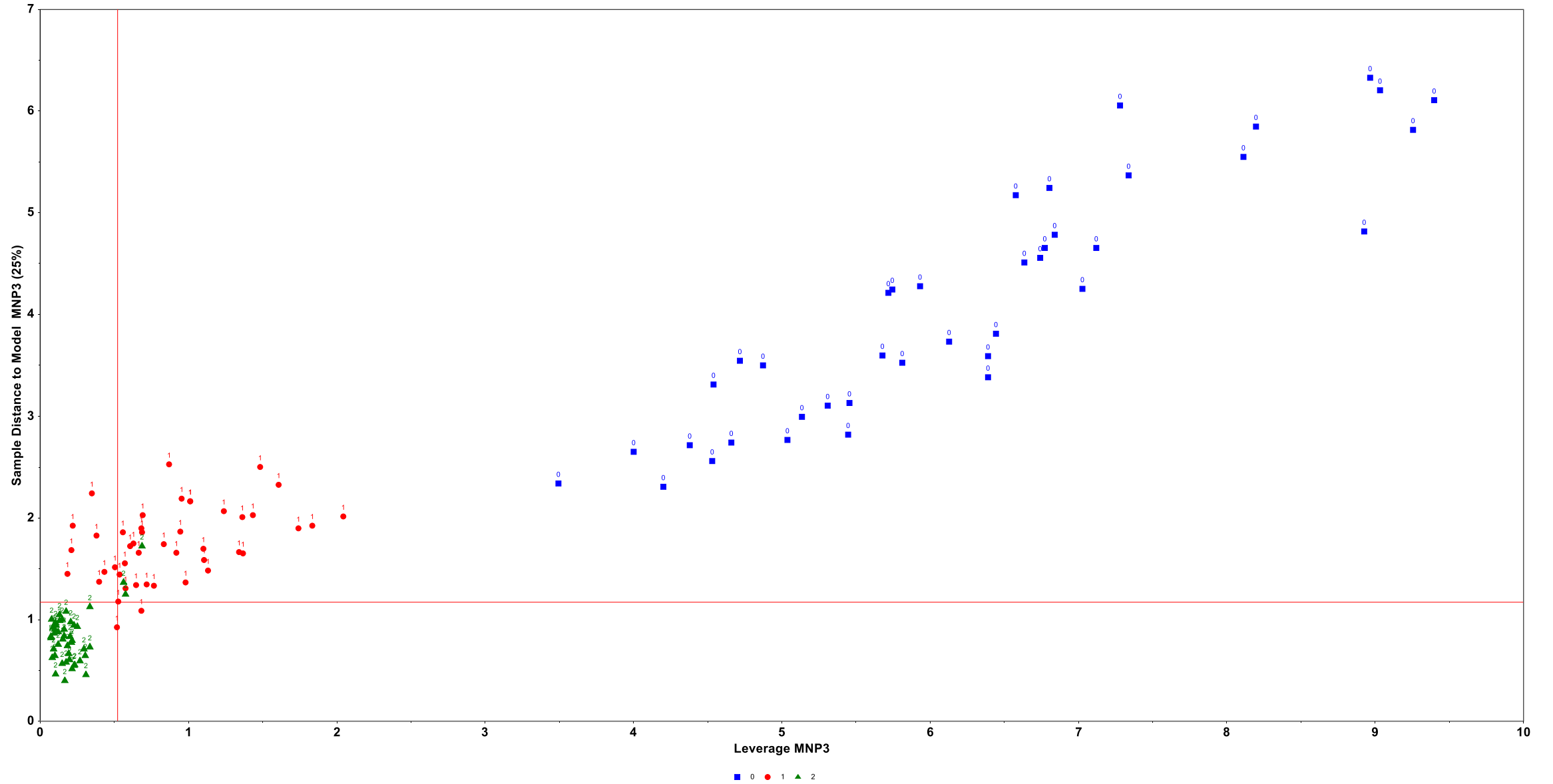
Si/S0 vs. Hi
