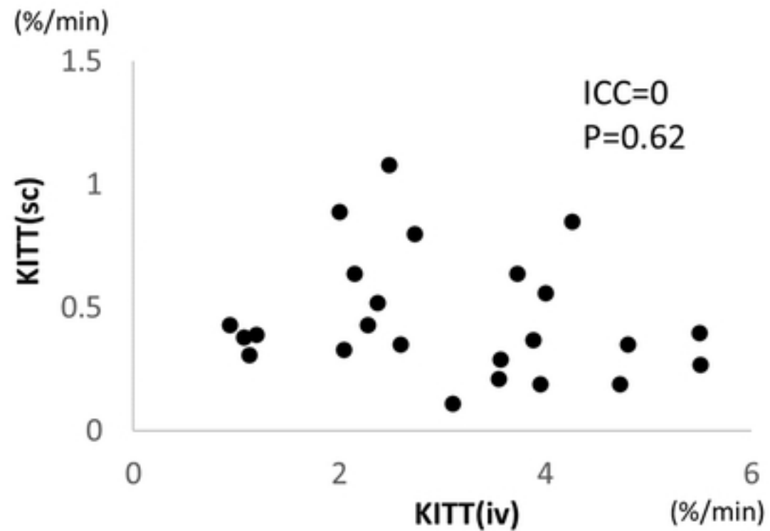
b. KITT(iv) vs KITT(sc)
