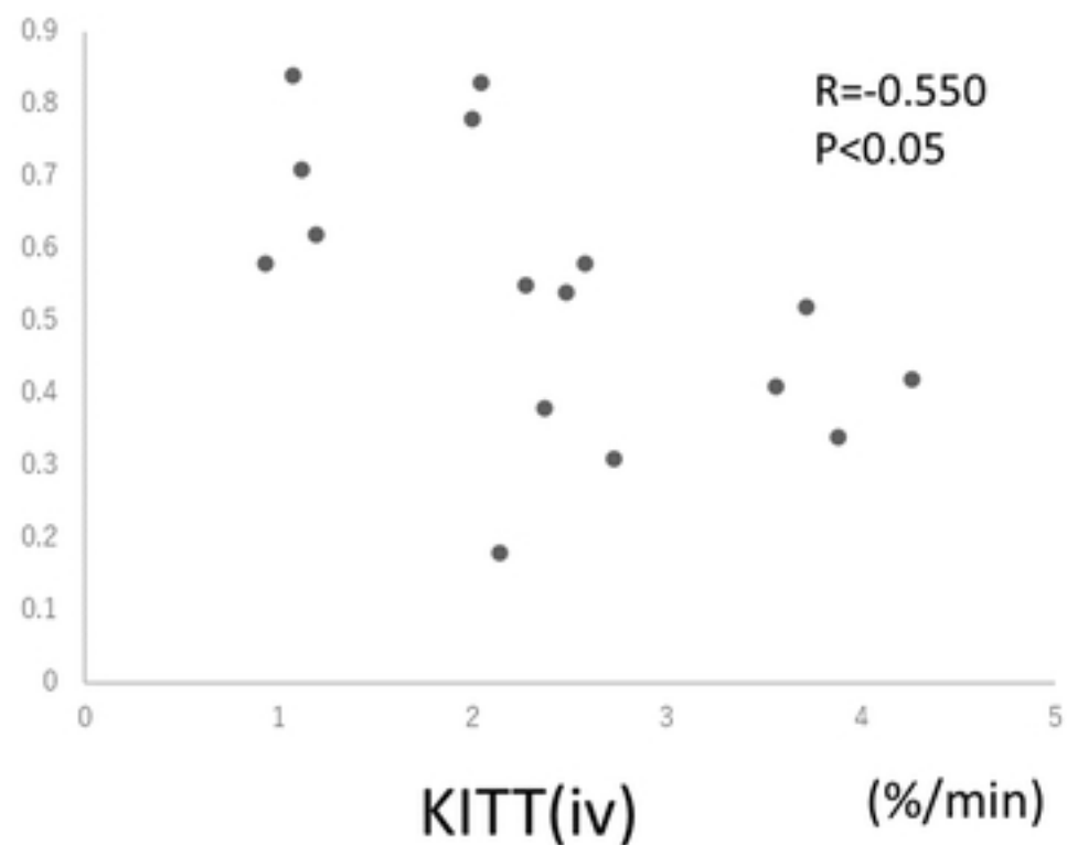
a. KITT(iv) vs mean total insulin dose/kg
