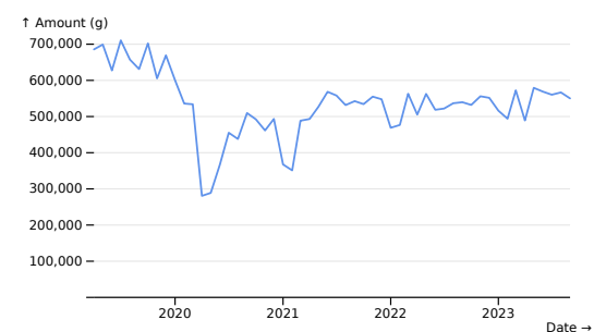
Ibuprofen
