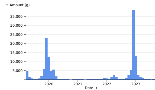
Oseltamivir phosphate
