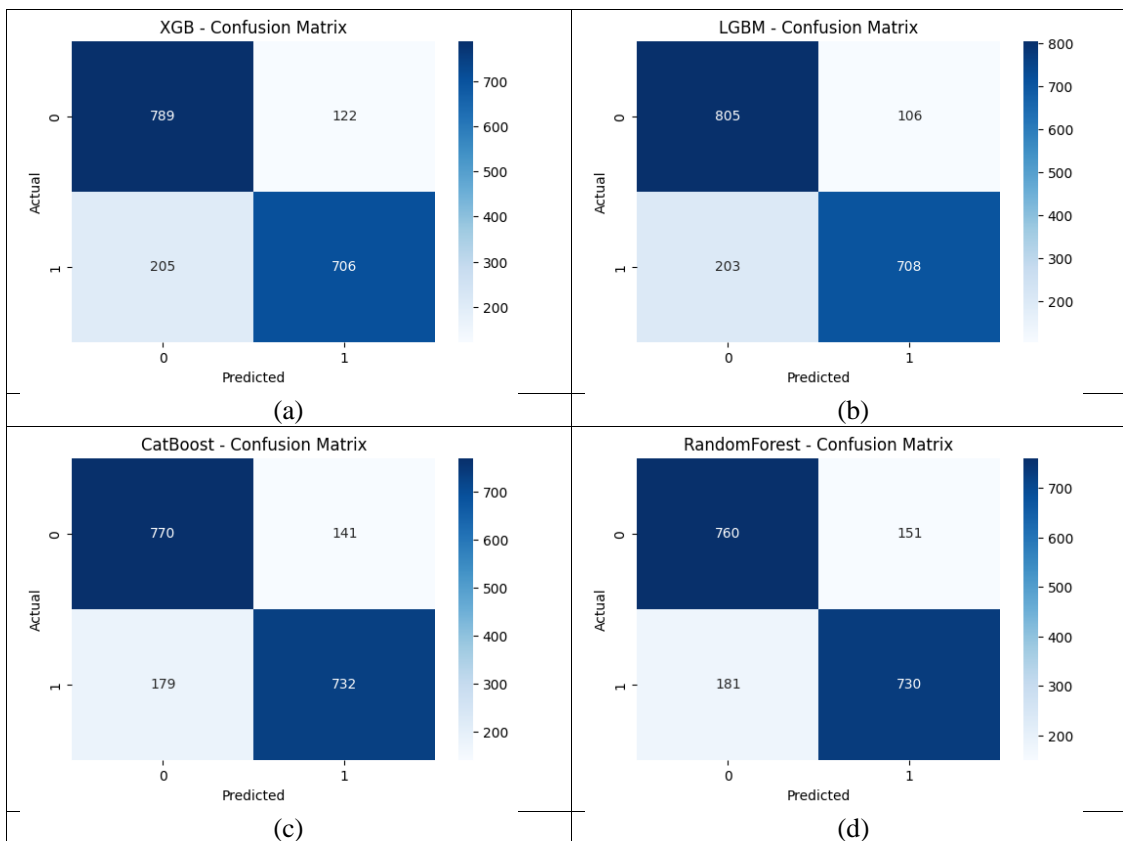
Figure 2. Confusion matrix: XGBoost (a), LGBM (b), CatBoost (c), RandomForest (d)
