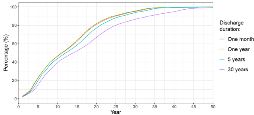
(b) ^{137}\text{Cs}
