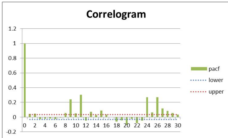
(d) PACF for death cases
