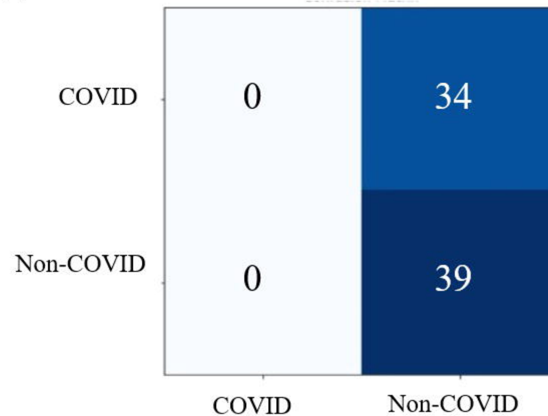
Inception V3
