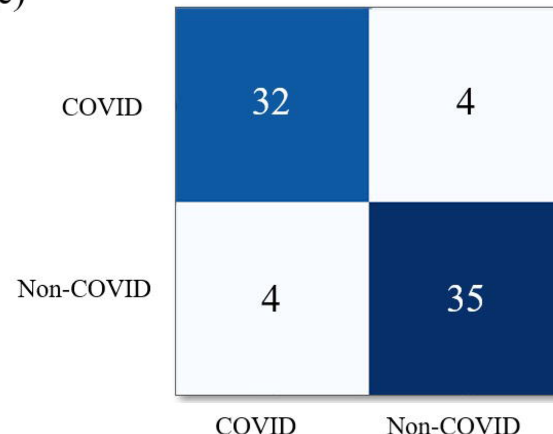
VGG-16
